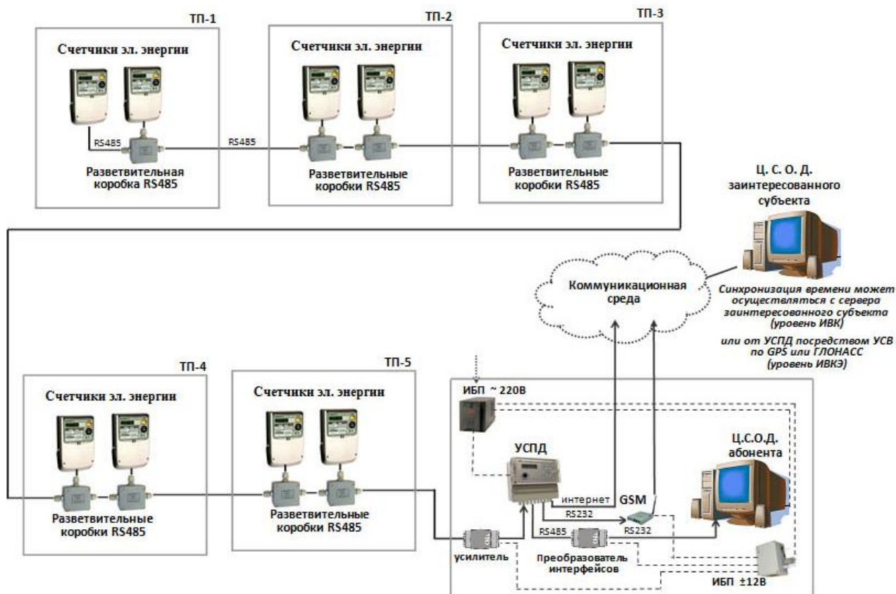
Рисунок 1 – Типовая схема организации АИИС КУЭ
