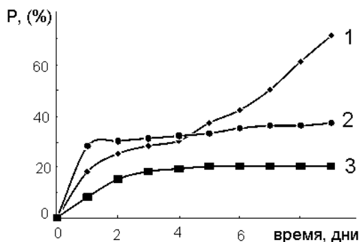
Рис. 2. Временная зависимость деструкции органического красителя под действием \text{H}_2\text{O}_2 в присутствии \text{CuFe}_2\text{O}_4 (1), \text{CoFe}_2\text{O}_4 (2), без катализатора (3)
