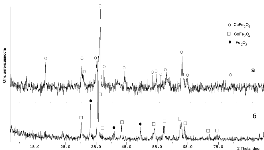
Рис. 1. Рентгенограммы образцов \text{CuFe}_2\text{O}_4 (а) и \text{CoFe}_2\text{O}_4 (б)
